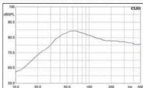
In knapp 40 Litern läuft der SX1 sehr harmonisch, die 44 Hz Einbauresonanz ermöglichen eine gute Tiefbassausbeute
