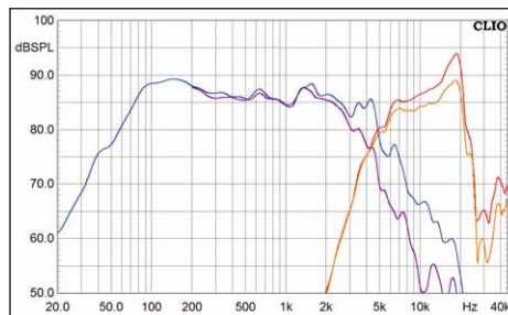
Der Tieftöner läuft ordentlich bis weit in den Mittelton, der Hochtöner wird sehr hoch eingekoppelt und rettet sich mittels der Membranresonanz bis an die 20-kHz-Marke
